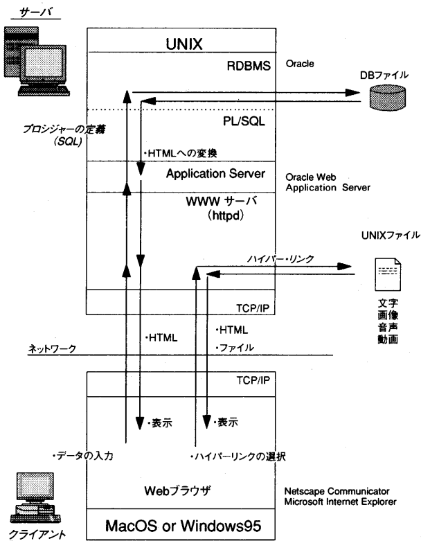
図2 システムソフトウェアの基本構成
